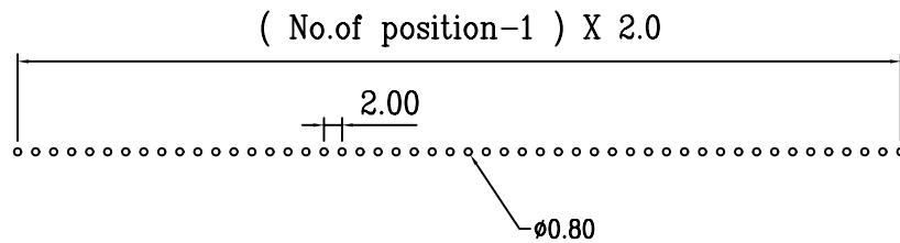
P.C.B.layout
