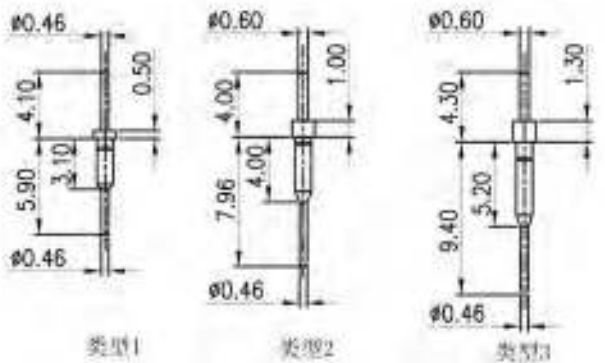
3种类型的端子尺寸公差为0.05
